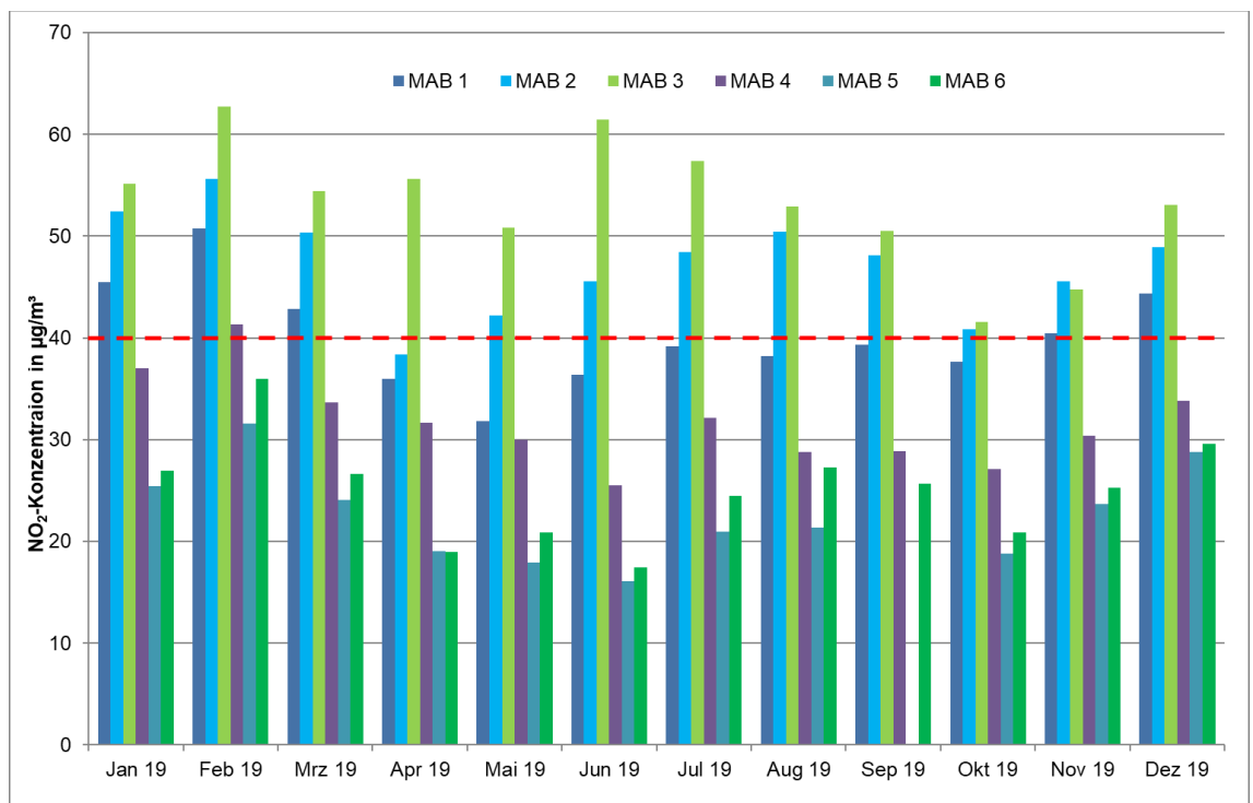
Abbildung 9. Verlauf der gemessenen NO 2 -Konzentrationen an den Messstandorten MAB-1 und MAB-6 für den Messzeitraum 02.01.19 - 03.01.20 (Monatsmittelwerte, NO 2 Grenzwert für das Kalenderjahr 40 µg/m 3 rot gestrichelt markiert).
