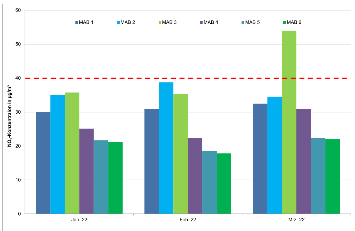
Abbildung 1. Verlauf NO 2 -Konzentration (Messzeitraum vom 03.01.2022 bis 02.04.2022).
